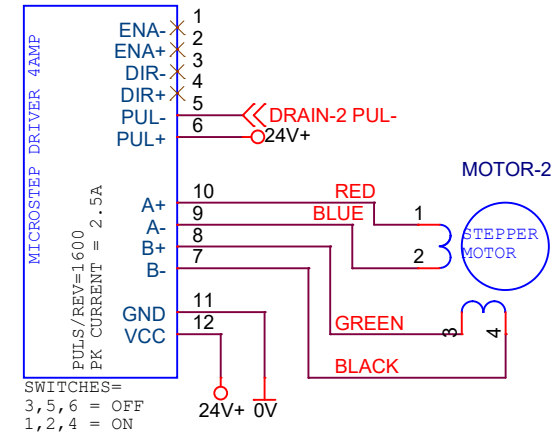
DRV-2
