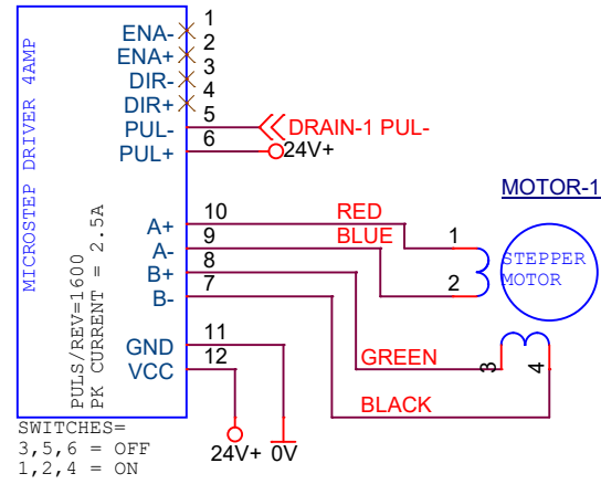
DRV-1
