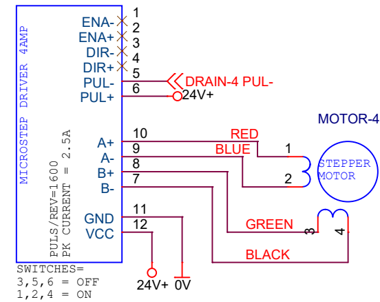
DRV-4
