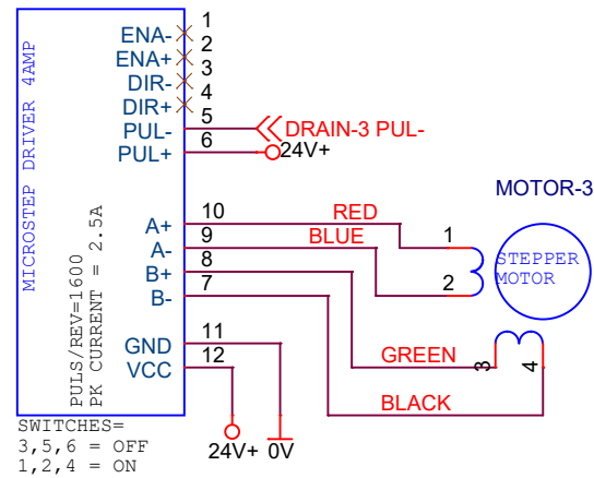
DRV-3
